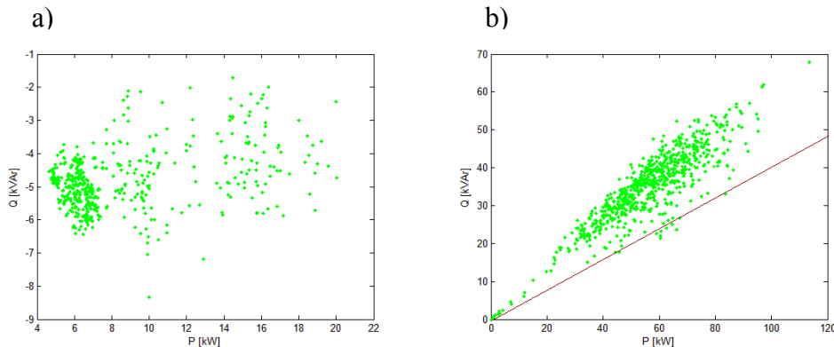
Rys. 2. Wykres rozrzutu pomiarów mocy czynnej P i biernej Q w punkcie zasilania odbiorów: budynku biurowego (a) i gospodarstwa ogrodniczego (b). Wartość ujemna Q świadczy o obciążeniu pojemnościowym, dodatnia – indukcyjnym. Linia prosta na rysunku b odpowiada relacji przy współczynniku mocy \operatorname{tg}\varphi = 0,4
