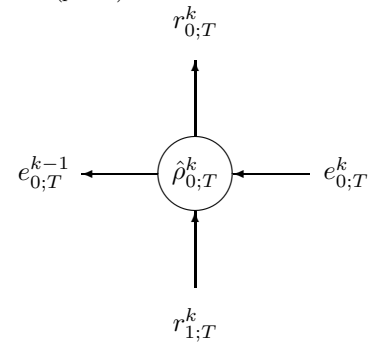
Fig. 8. Schur parametrization ( p = 2 ).
