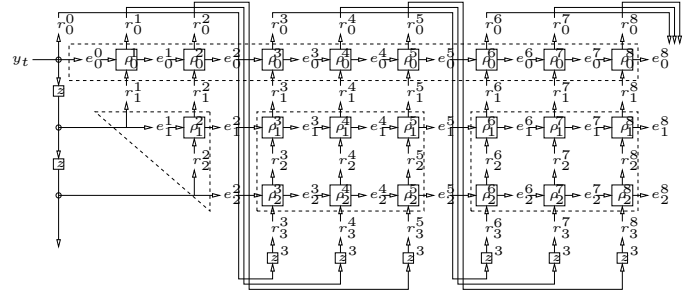
Fig. 8. Schur parametrization ( p = 2 ).
