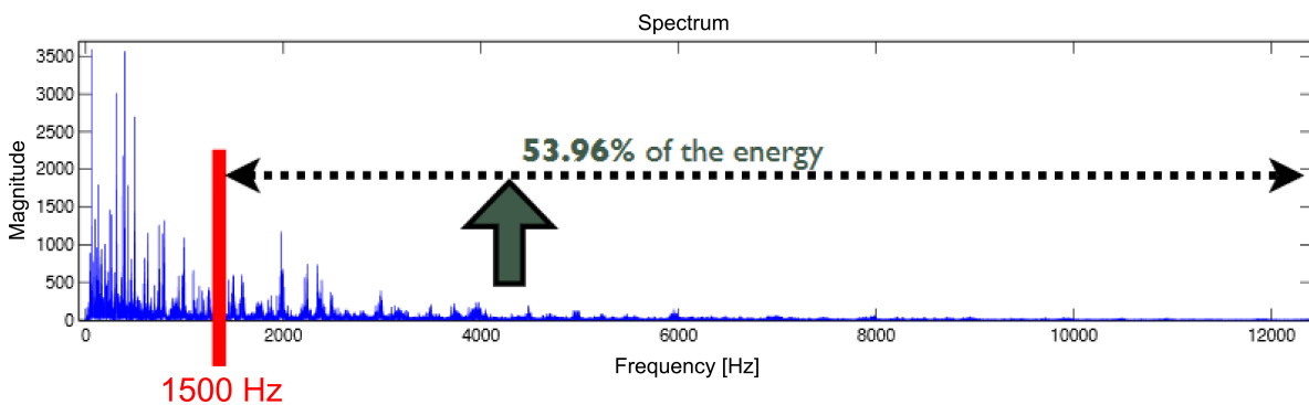
Fig. 3. Brightness (MIRtoolbox).
