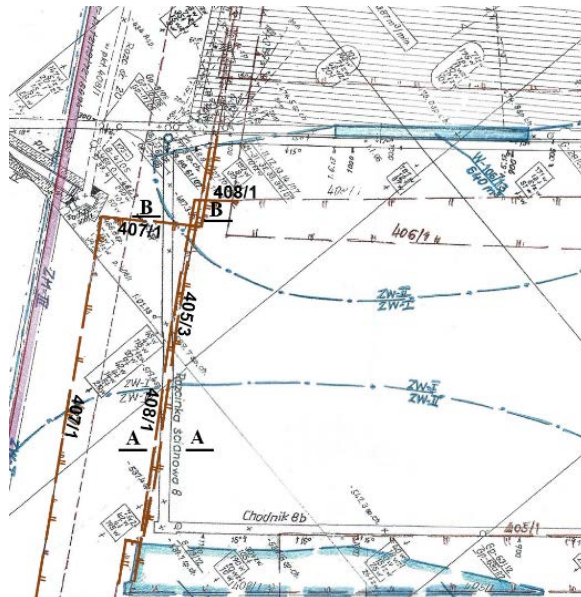
Rys. 12. Wycinek mapy pokładu 408/2 z naniesioną rozciną ścianową 8 i zaznaczonymi zaszłościami eksploatacyjnymi (Bobek in. 2013)
