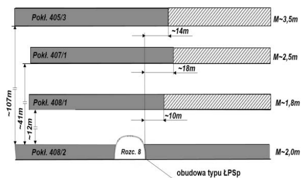
Rys. 13. Przekrój B-B – usytuowanie krawędzi pokładów względem rozcinu ścianowej 8 w pokładzie 408/2 (Bobek i in. 2013)
