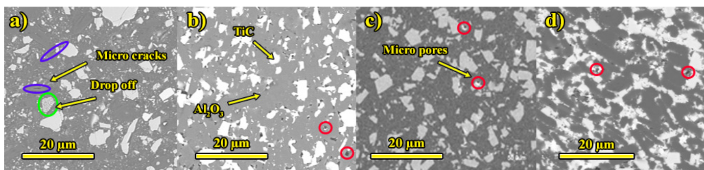
Fig. 6. FESEM of the composites a) 20% b) 25% c) 30% d) 35% TiC
