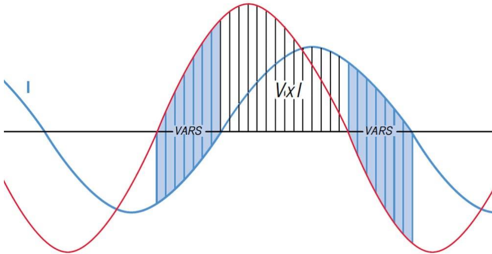
Fig. 1. \cos\varphi or DPF
