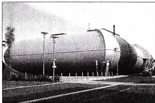
Fot. 1. „Trudelturm” przed Instytutem Chemii (powyżej) oraz Wielki Kanał Wiatrowy (poniżej).
