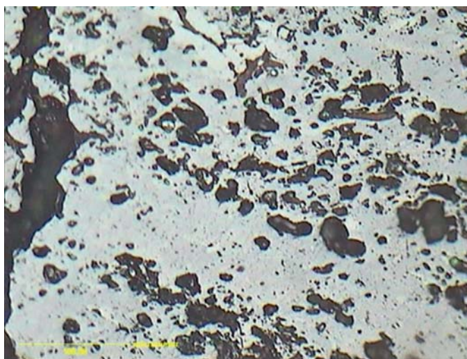
Fot. 3. Węgiel przeobrażony termicznie pod wpływem pożaru zwałowiska. Widoczne liczne pory powstałe w wyniku odgazowania. Światło odbite, obiektyw imersyjny, pow. 200×
