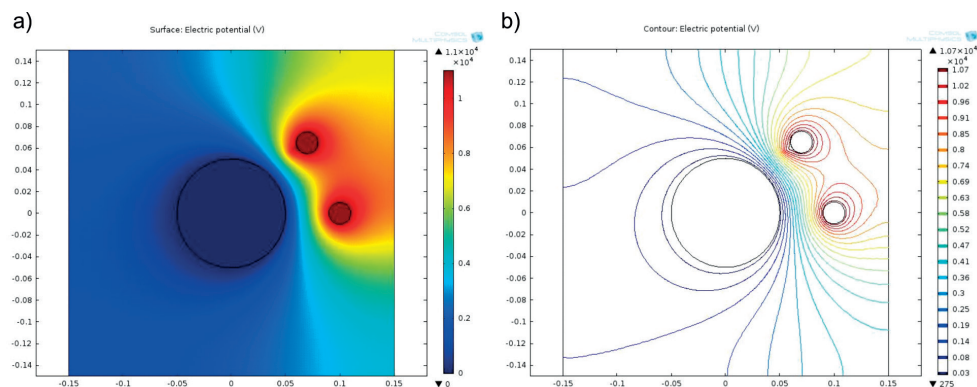
Rys. 8. Rozkład potencjału elektrycznego w układzie analizowanego separatora a) rozkład powierzchniowy, b) linie potencjału elektrycznego
