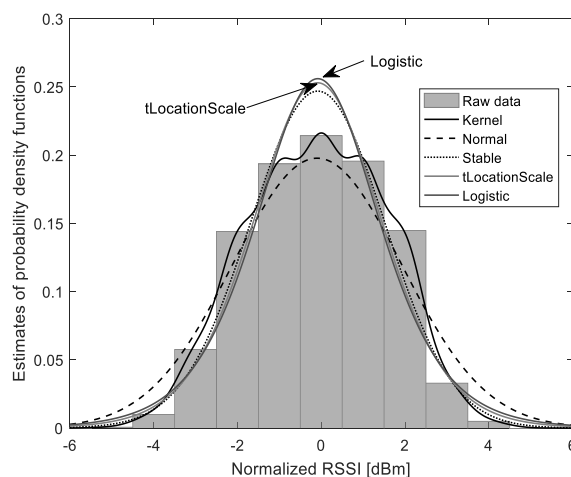
Fig. 5. PDF estimates for 2.4 GHz band (ESP 8266).
