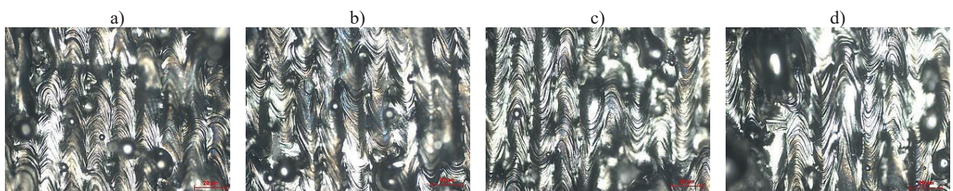
Fig. 6. Light microscope images represents the differences of SLM parts made: (a) h=25\ \mu\text{m} , t=25\ \mu\text{s} ; (b) h=25\ \mu\text{m} , t=100\ \mu\text{s} ; (c) h=100\ \mu\text{m} , t=25\ \mu\text{s} ; (d) h=100\ \mu\text{m} , t=100\ \mu\text{s} ; mag. 1000x
