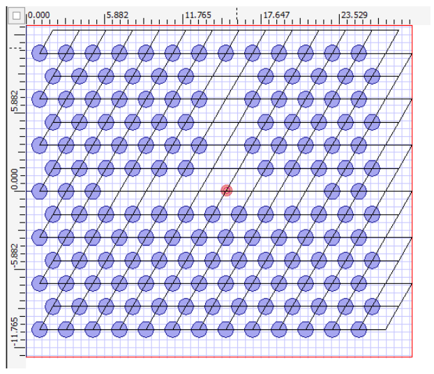
Fig. 1 (d). PCF structure D
