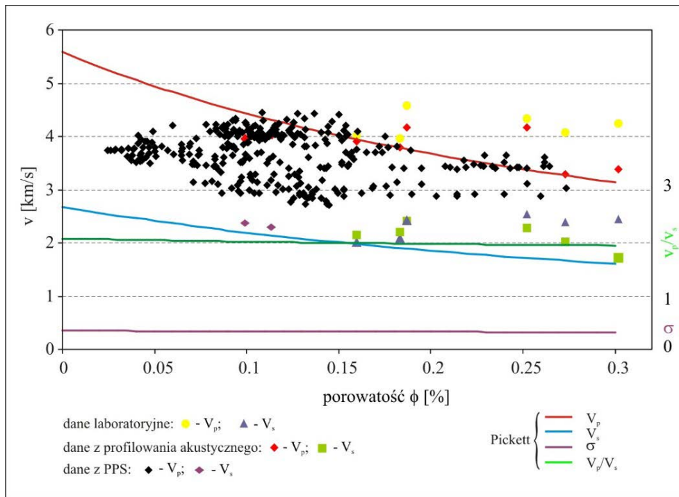
Rys. 3. Zestawienie zależności pomiędzy parametrami petrofizycznymi złoża siarki według formuły Picketta z danymi różnych metod pomiarowych
