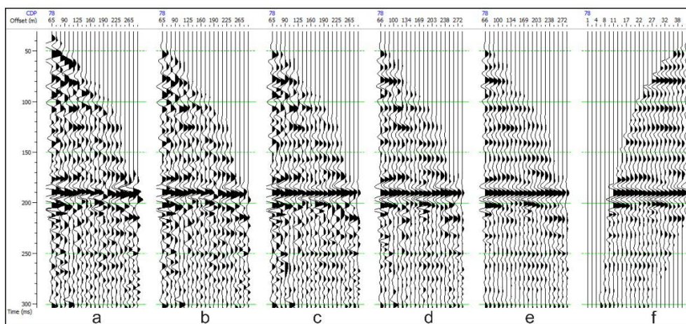
Rys. 2. Zestawienie wyników kolejnych etapów przetwarzania dla celów inwersji sejsmicznej: a) kolekcja CMP, b) filtracja pasmowa, c) statyka resztkowa, d) super kolekcja, e) transformacja Radona, f) kolekcja kątowna
