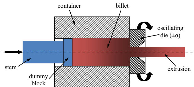
Fig. 1. Schematic of die rotation oscillating extrusion
