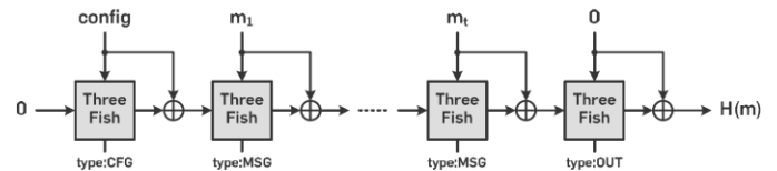
Fig. 7. Skein normal hashing scheme
