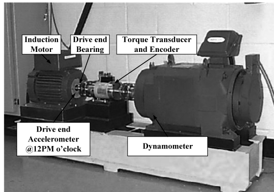
Fig. 3. Experimental test rig.
