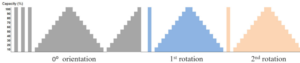
Fig. 1. Calibration procedure D.1 in DIN 51309.
