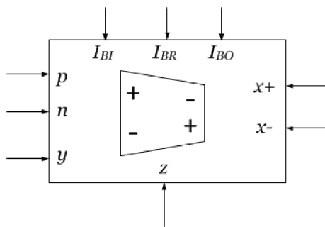
Fig. 4. MCDTA symbol
