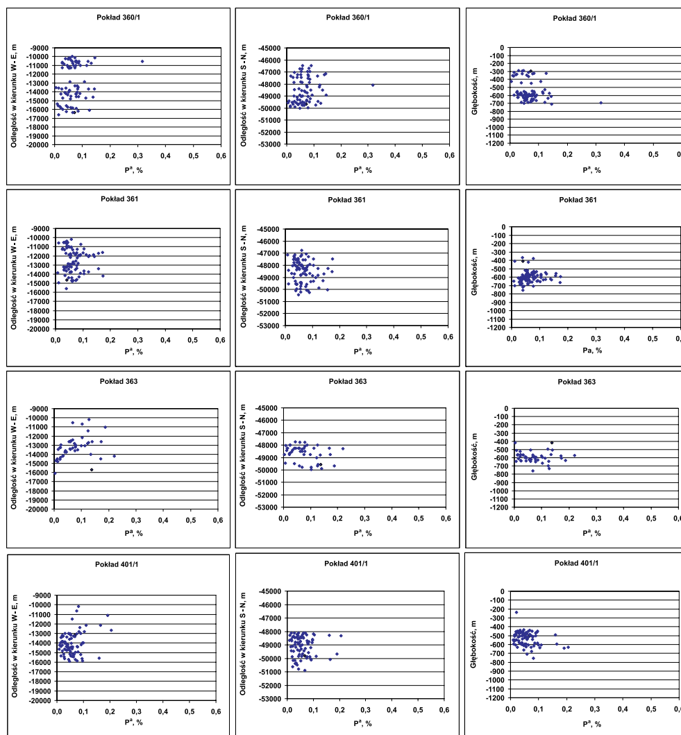
Rys. 4. Zmiany zawartości fosforu w badanych pokładach w ujęciu horyzontalnym i wertykalnym. Objasnienie jak na rysunku 3; pokazano jedynie pokłady, gdzie liczba próbek była wyższa od 30.
