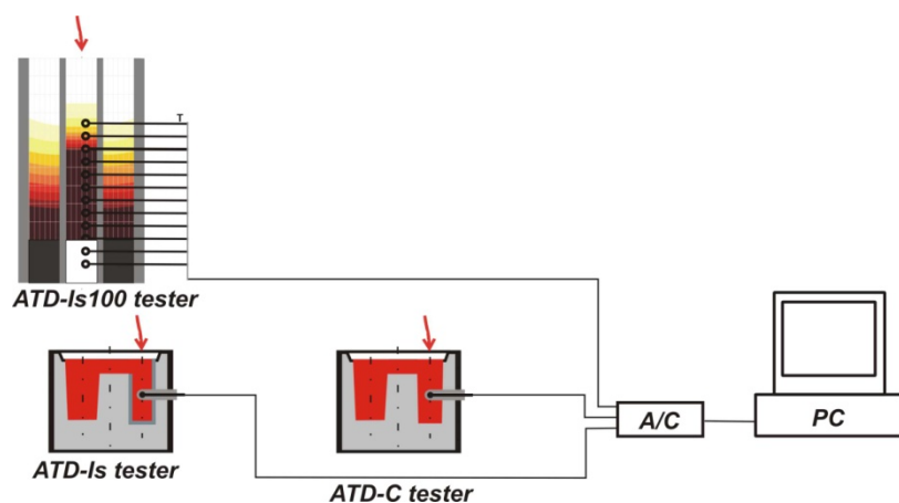
Fig. 1. Test stand
