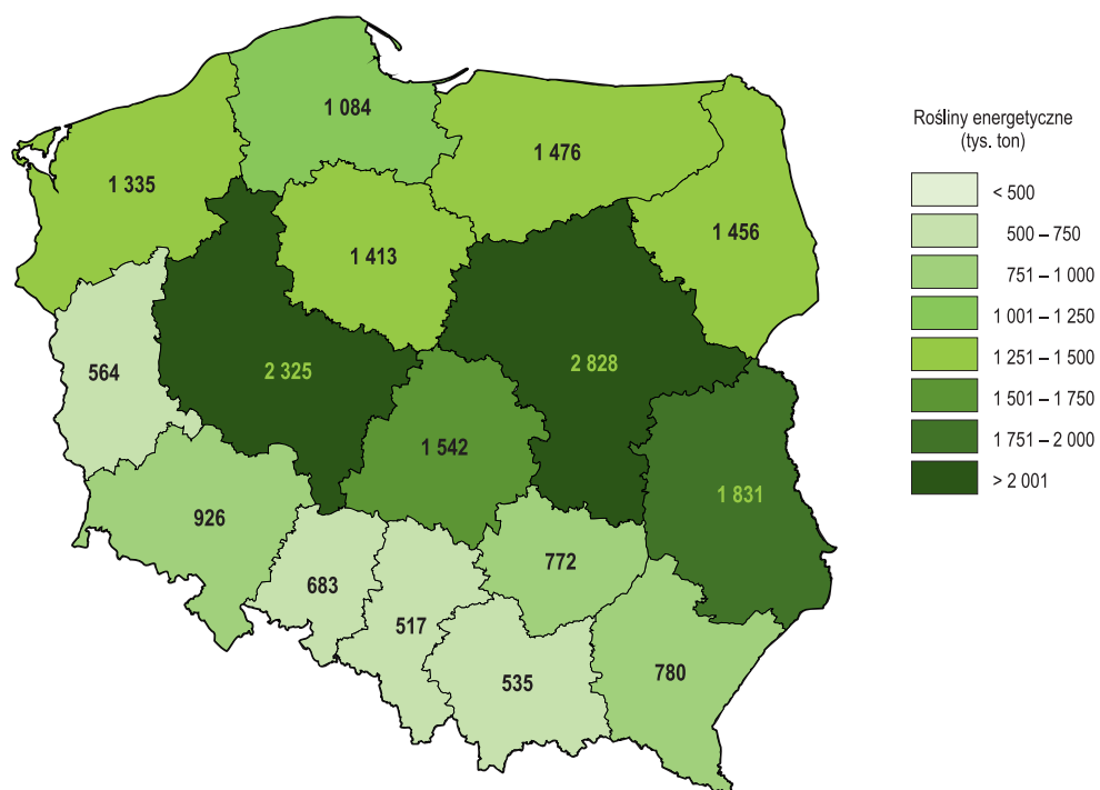
Ryc. 4. Potencjał techniczny biomasy stałej z wieloletnich plantacji roślin energetycznych. Źródło: Instytut Uprawy, Nawożenia i Gleboznawstwa; [Jasiulewicz 2010].
